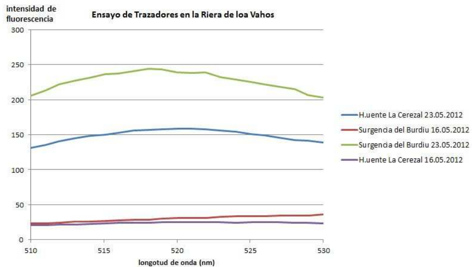
Figura 3.-Resultados del fluorímetro para cada captador de carbono activo.
